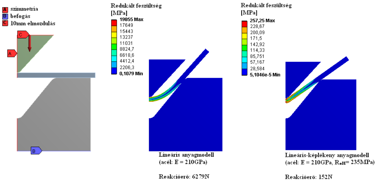
2.15. ábra: Rugalmas és képlékeny anyagmodell alkalmazása
